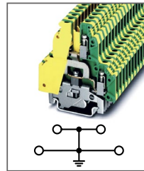
RUKK 5-PE
