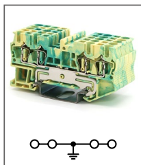
RNS 2,5-QUOTTRO-PE
